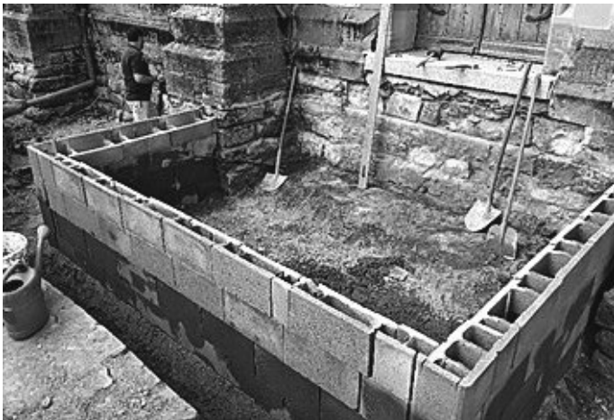
Beton-Schalensteine bilden den äußeren Kranz des Fundaments
